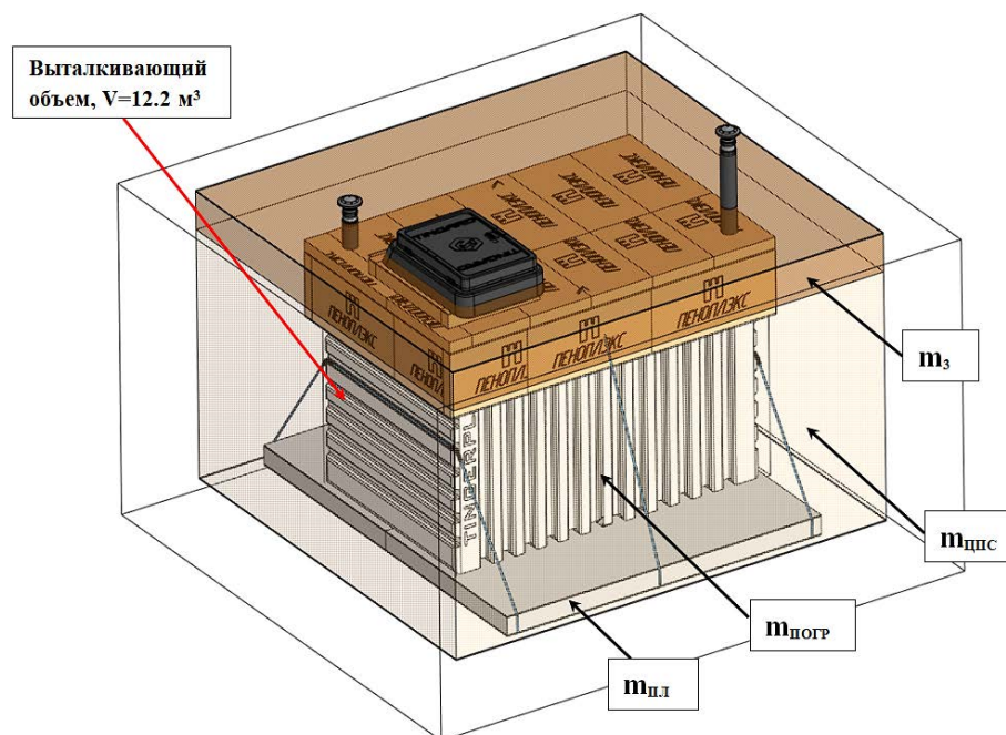
Рисунок 11 – Расчет якорения погреба
