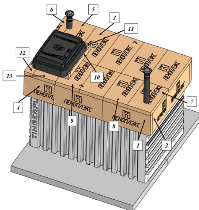
Рисунок 8 – Схема монтажа утеплителя
