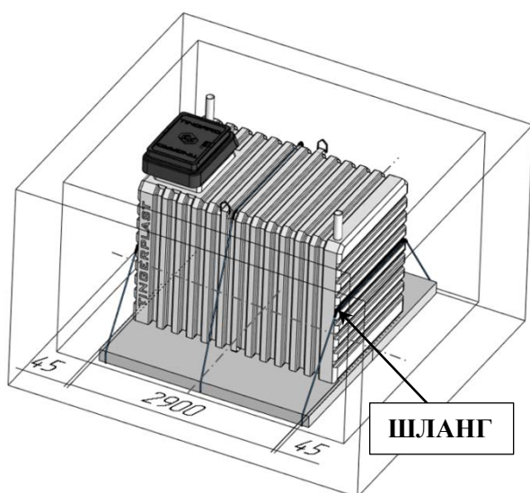
Рисунок 4 – Установка погреба
