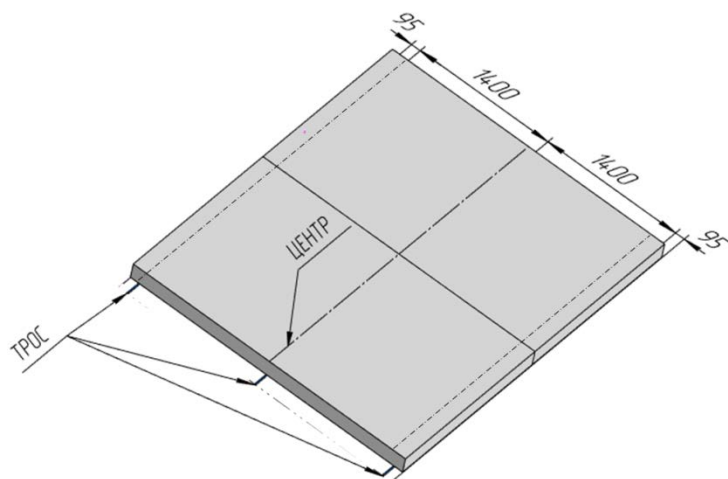
Рисунок 2 – Закладка тросов
