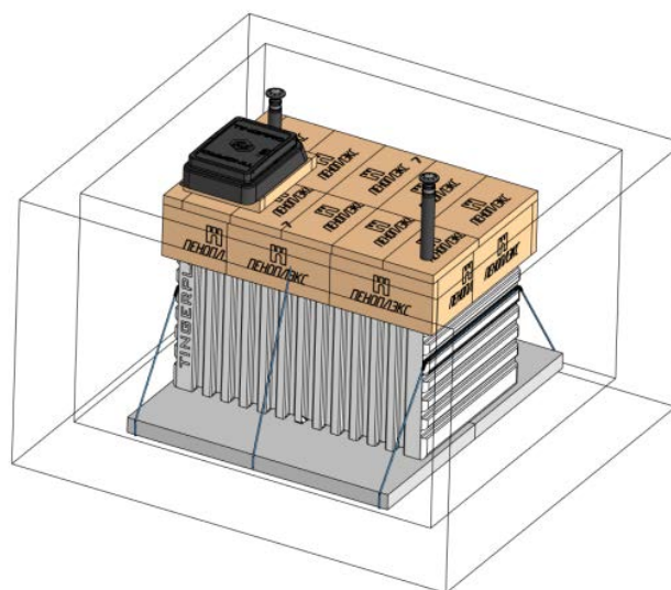
Рисунок 5 – Утепление погреба и закрепление тросами
